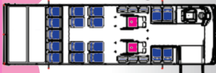
34', 9+24 Passenger, 6 w/c
