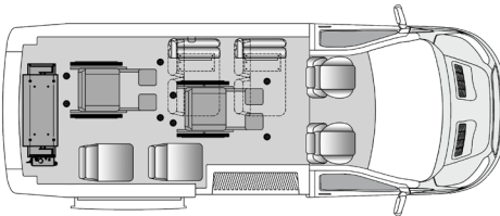
Essieu simple - Élévateur à l'arrière, 8 passagers plus deux fauteuils roulants
