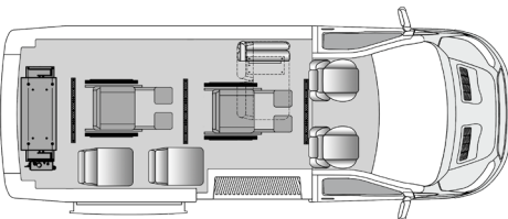
Essieu simple - Élévateur à l'arrière, 6 passagers plus deux fauteuils roulants
