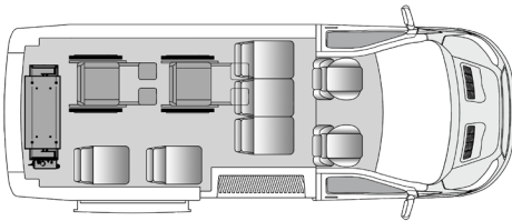
Essieu simple - Élévateur à l'arrière, 7 passagers plus deux fauteuils roulants
