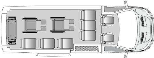
Essieu simple - Élévateur à l'arrière, 8 passagers plus deux fauteuils roulants
