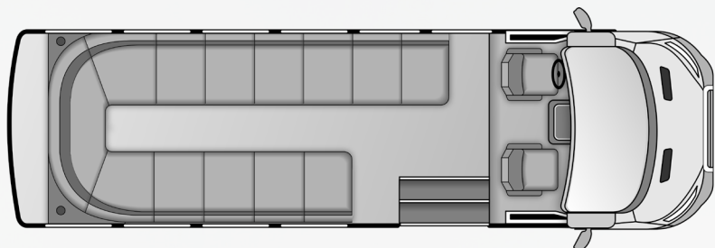
SALON 15 PASSAGERS (13+2)
